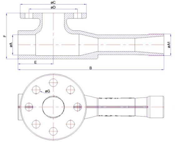
Ventüri Krokisi
